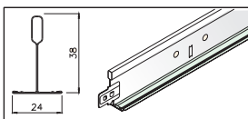
Tverrprofil
