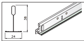
Hovedprofil
