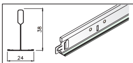
Hovedprofil
