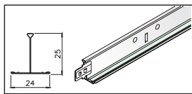
Tverrprofil
